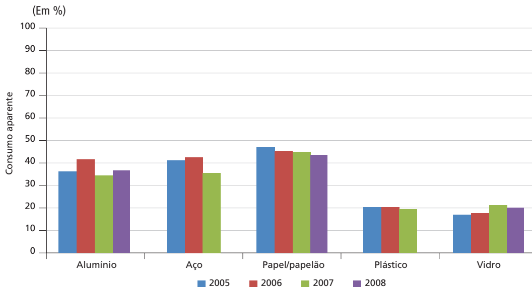
GRÁFICO 4 Taxa de reciclagem de diferentes materiais
